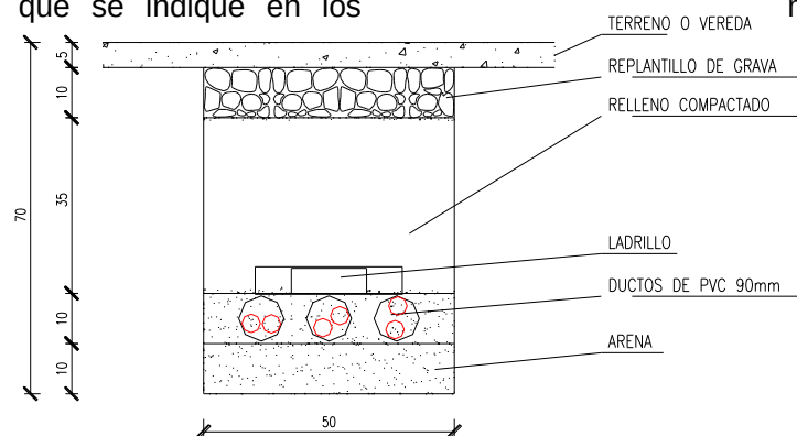
ZANJA TIPO 4
