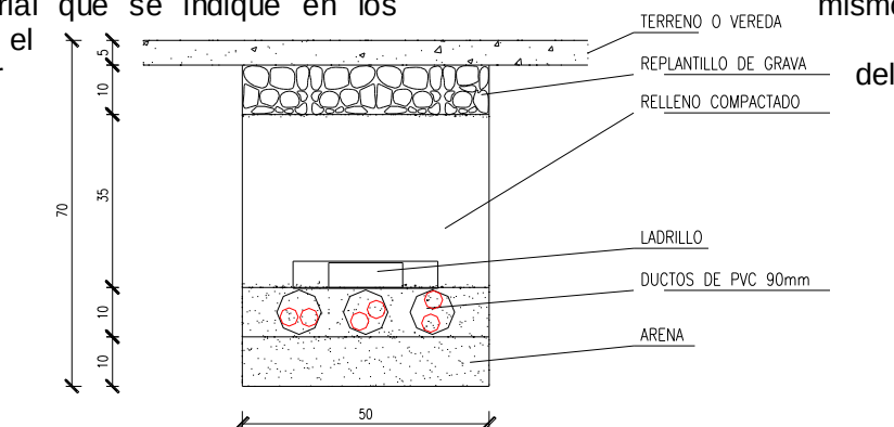
ZANJA TIPO 4
