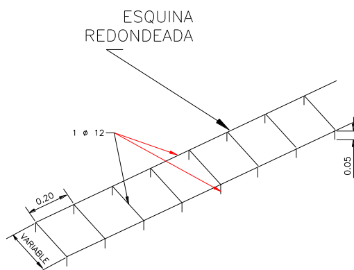
DETALLE DE PARRILLA METALICA
