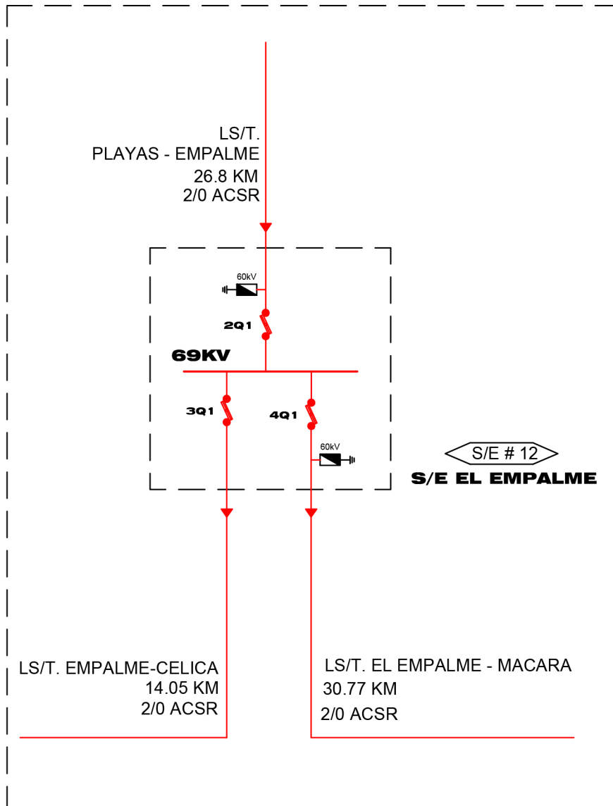
S/E # 12 S/E EL EMPALME ACTUAL
