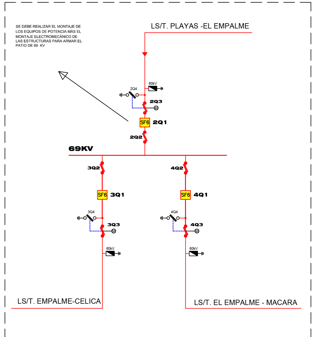
S/E # 12 S/E EL EMPALME PROYECTADA
